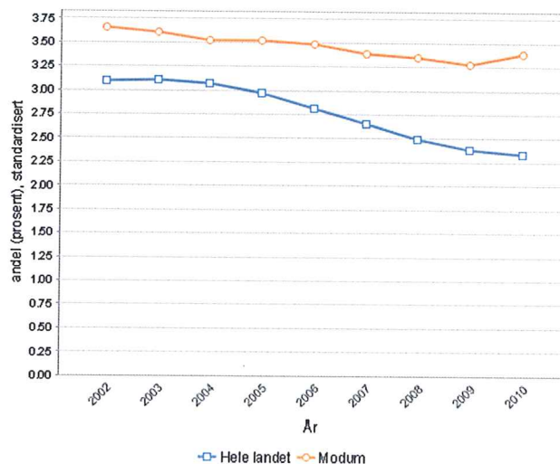
Figur 2. Uføretryggede under 45 år, 2002-2010
