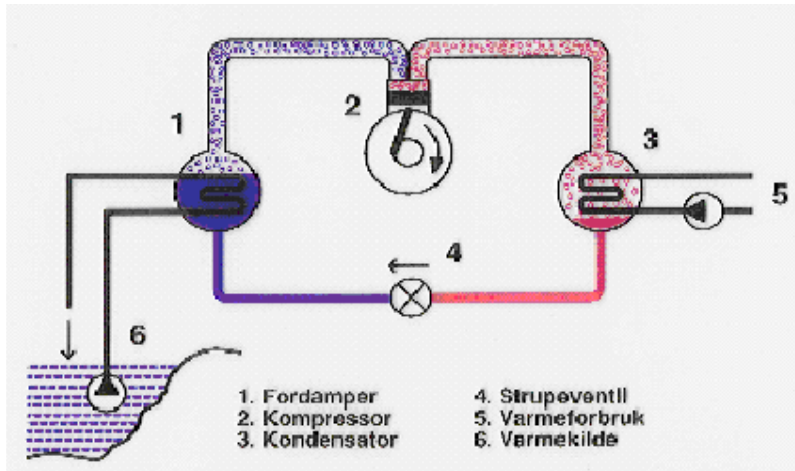
Figur 4. Prinsippskisse varmepumpe
